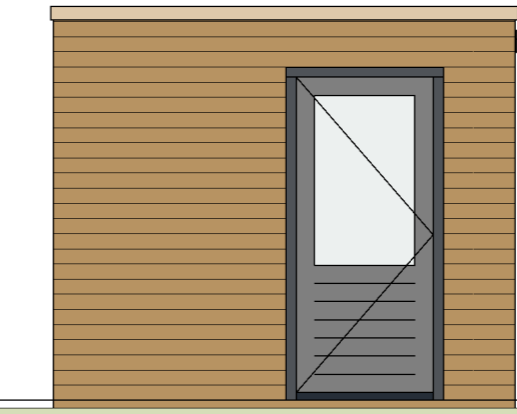
linkerzijgevel 1:50
