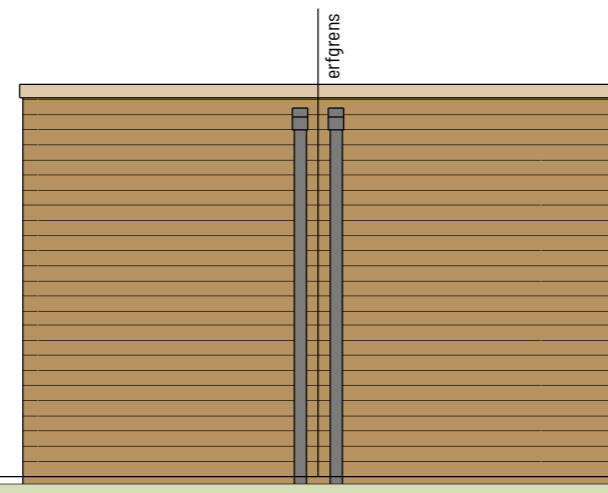
voorgevel 1:50
