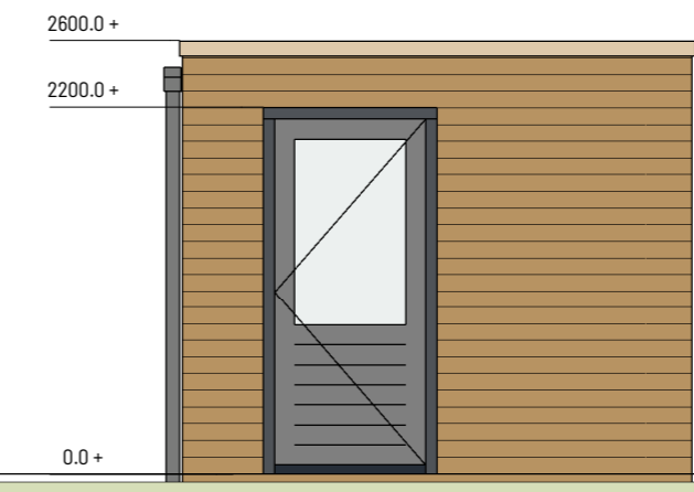
rechterzijgevel 1:50
