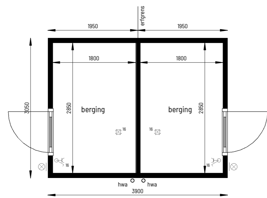
begane grond 1:50
