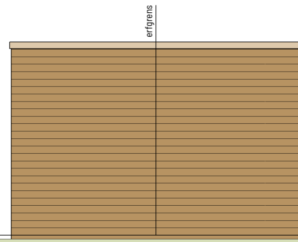
achtergevel 1:50
