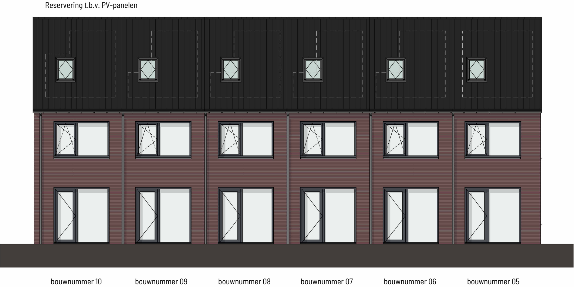
achtergevel
